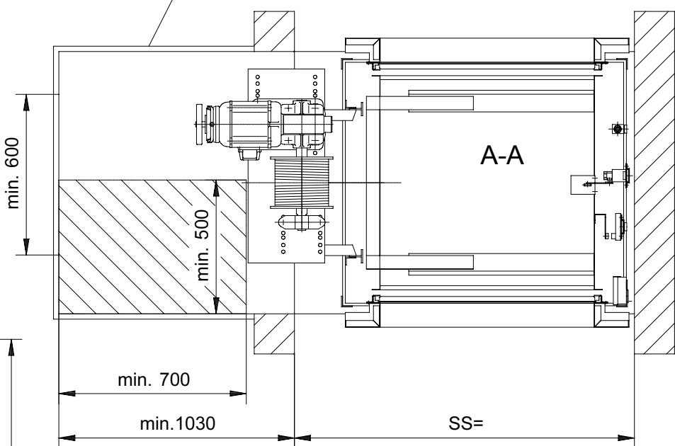
Obudowa i drzwi do maszynowni po stronie budowlanej
